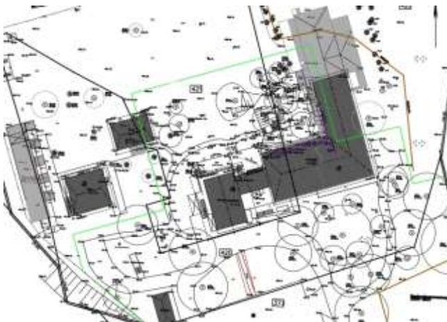
Beispiel Vermesserplan
